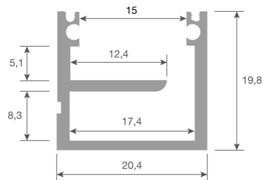
Maßstab 2:1
